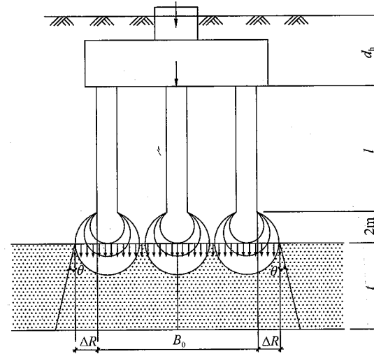
图 4.2.5 软弱下卧层计算示意
