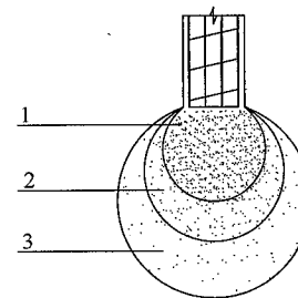
图1 填料载体构造 1—水泥砂拌合物；2—挤密土体；3—影响土体
