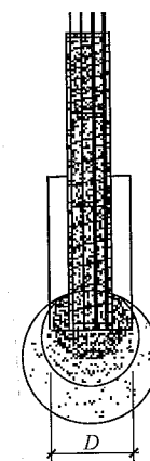
图 4.3.2 抗拔载体桩计算简图
